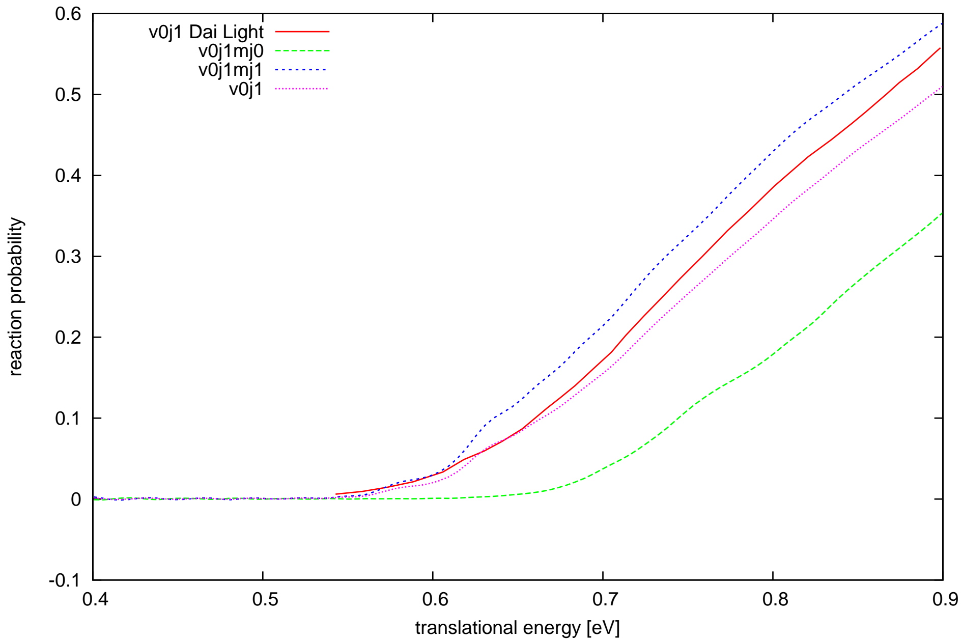
6D QD Dai Zhang LEPS PES v0j1
