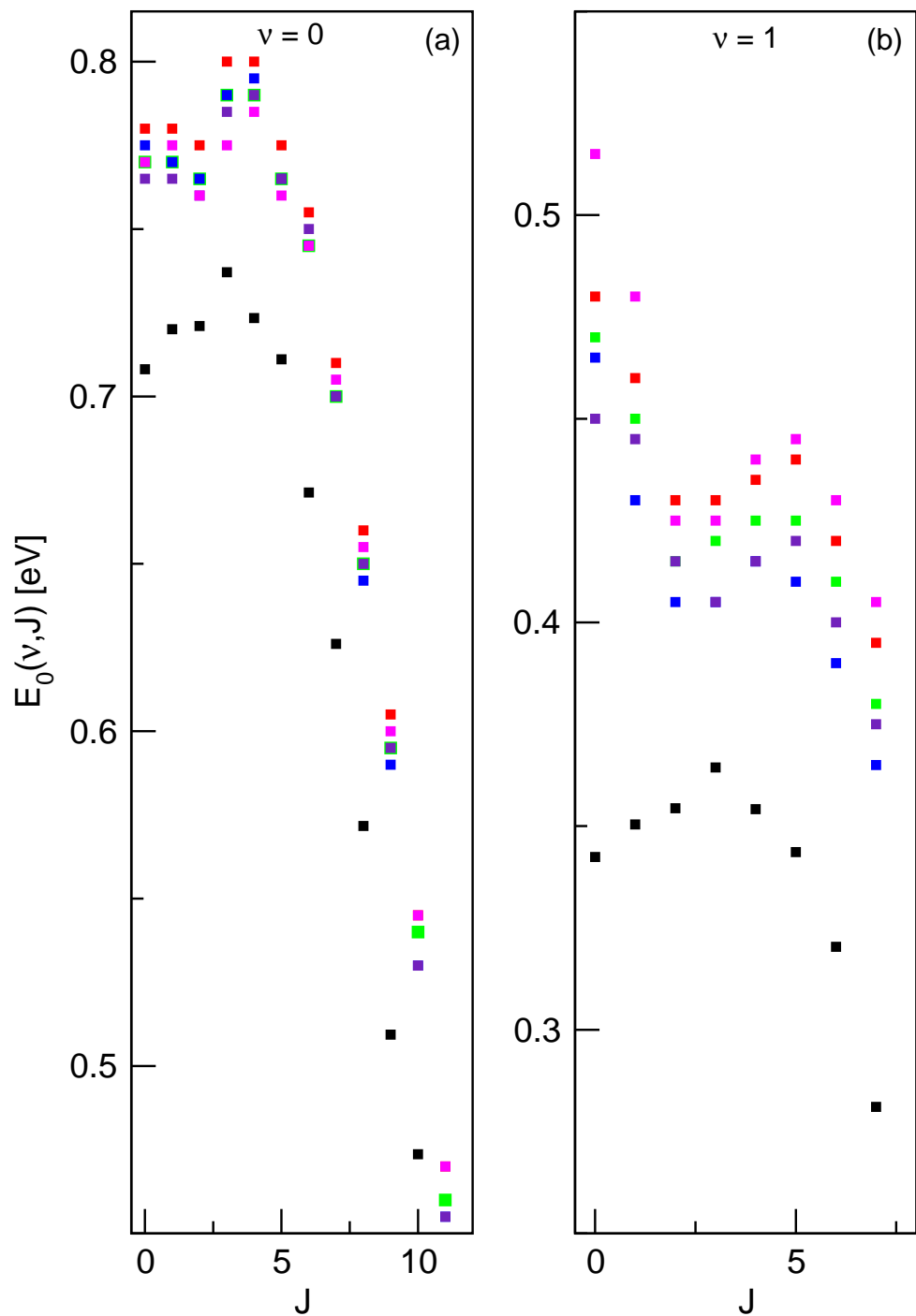
\text{H}_2 + \text{Cu}(111)
